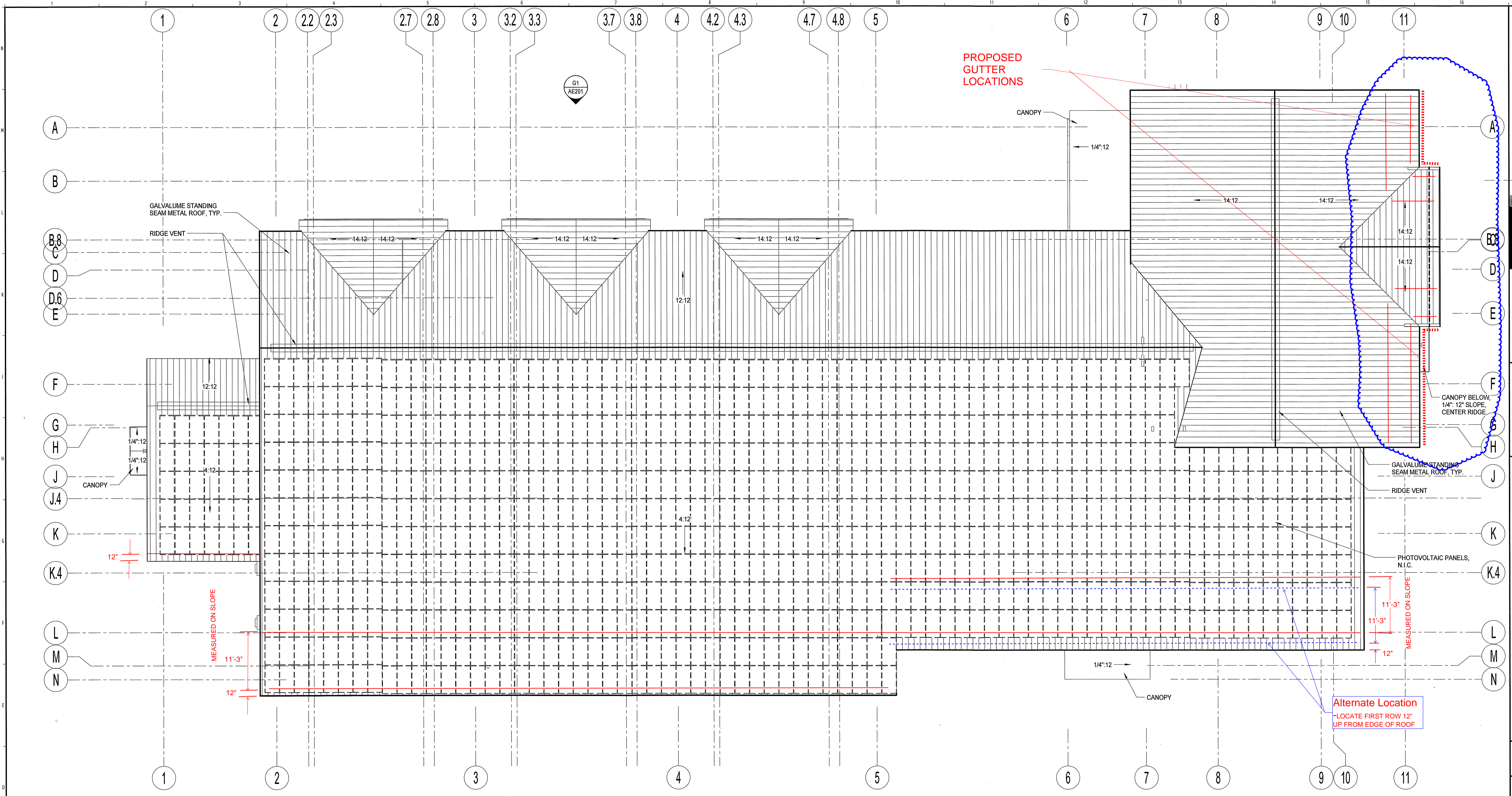
D1 ROOF PLAN 1/8" = 1'-0"
